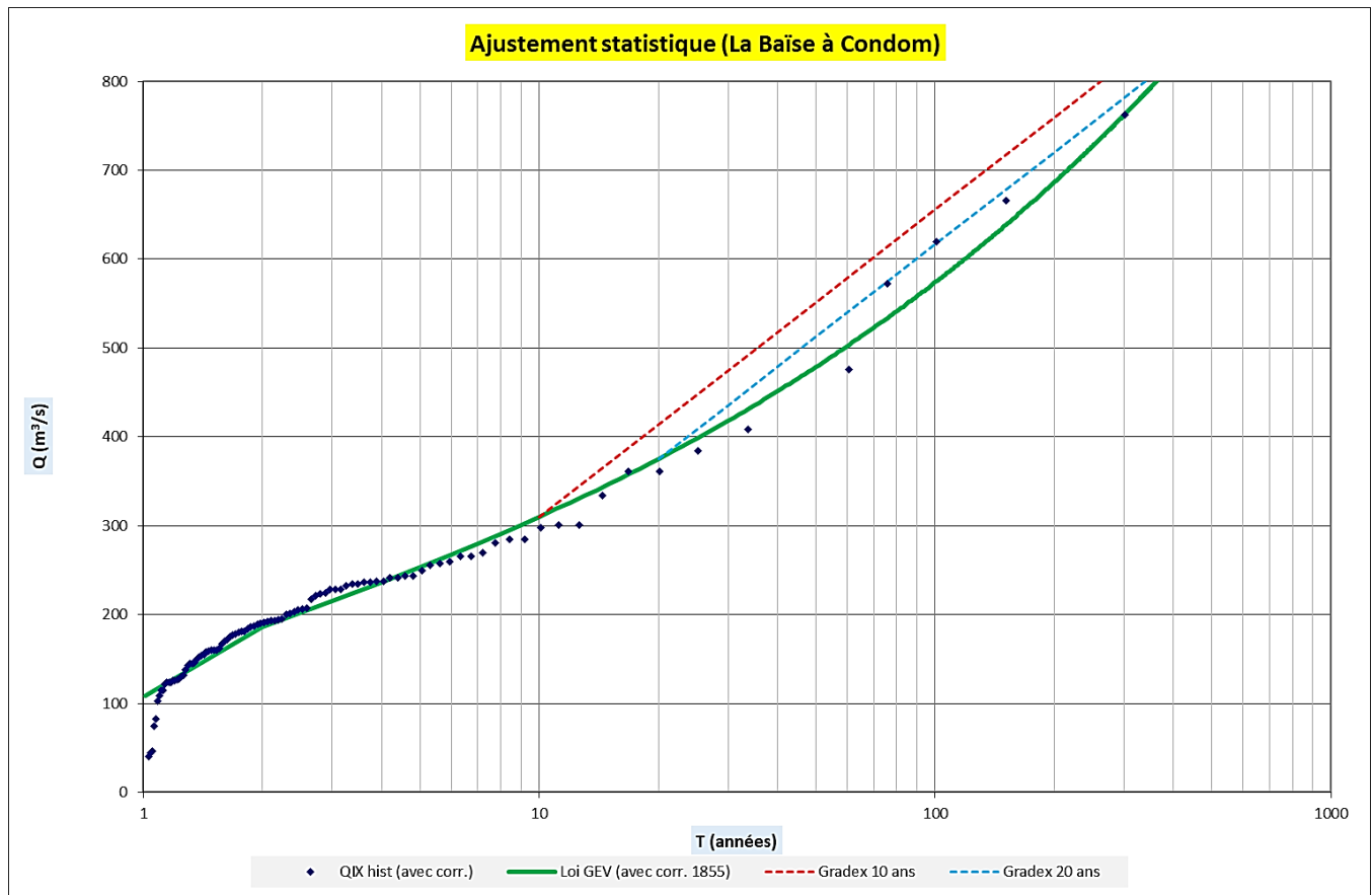
Figure 6 : Analyse fréquentielle des débits de crue pour la Baïse à Condom
