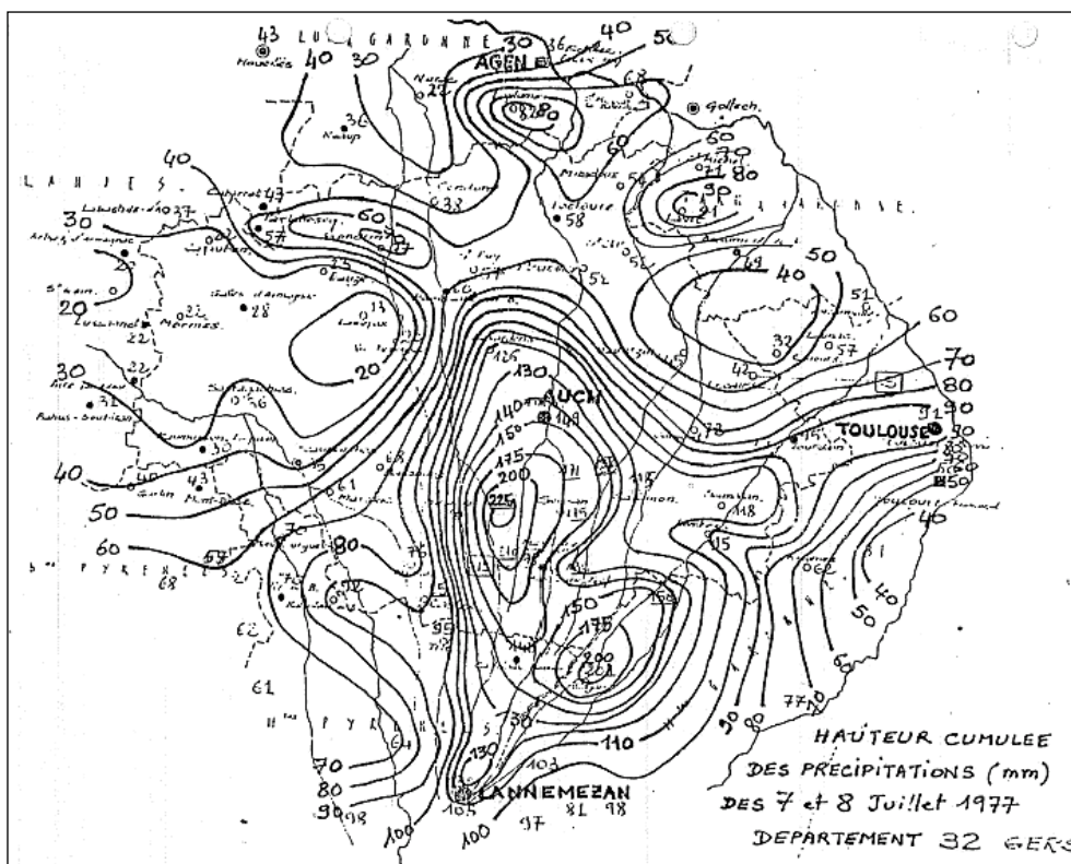
Figure 2 : Courbes isohyètes pour la pluie du 7 au 8 juillet 1977
