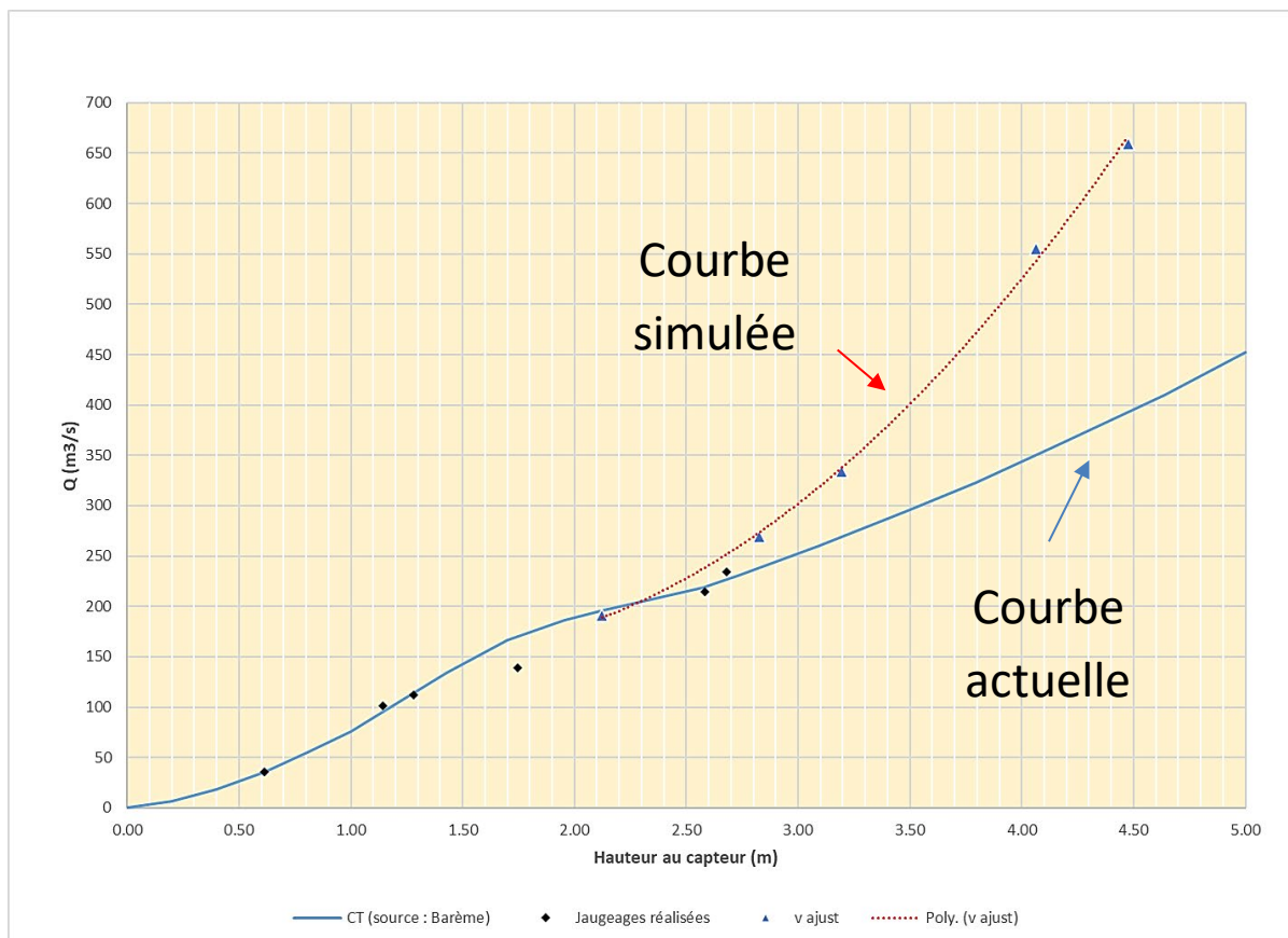
Figure 5 : Exemple de la courbe de tarage à Condom
