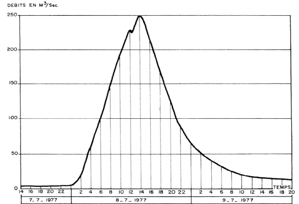
FIG. 4 Hydrogramme de la crue du Gers, à Pannasac, le 8 juillet 1977. Source : M. GAYRAUD et G. LALANNE, La crue du 8 juillet 1977 en Gascogne. Coteaux de Gascogne, octobre 1977.
