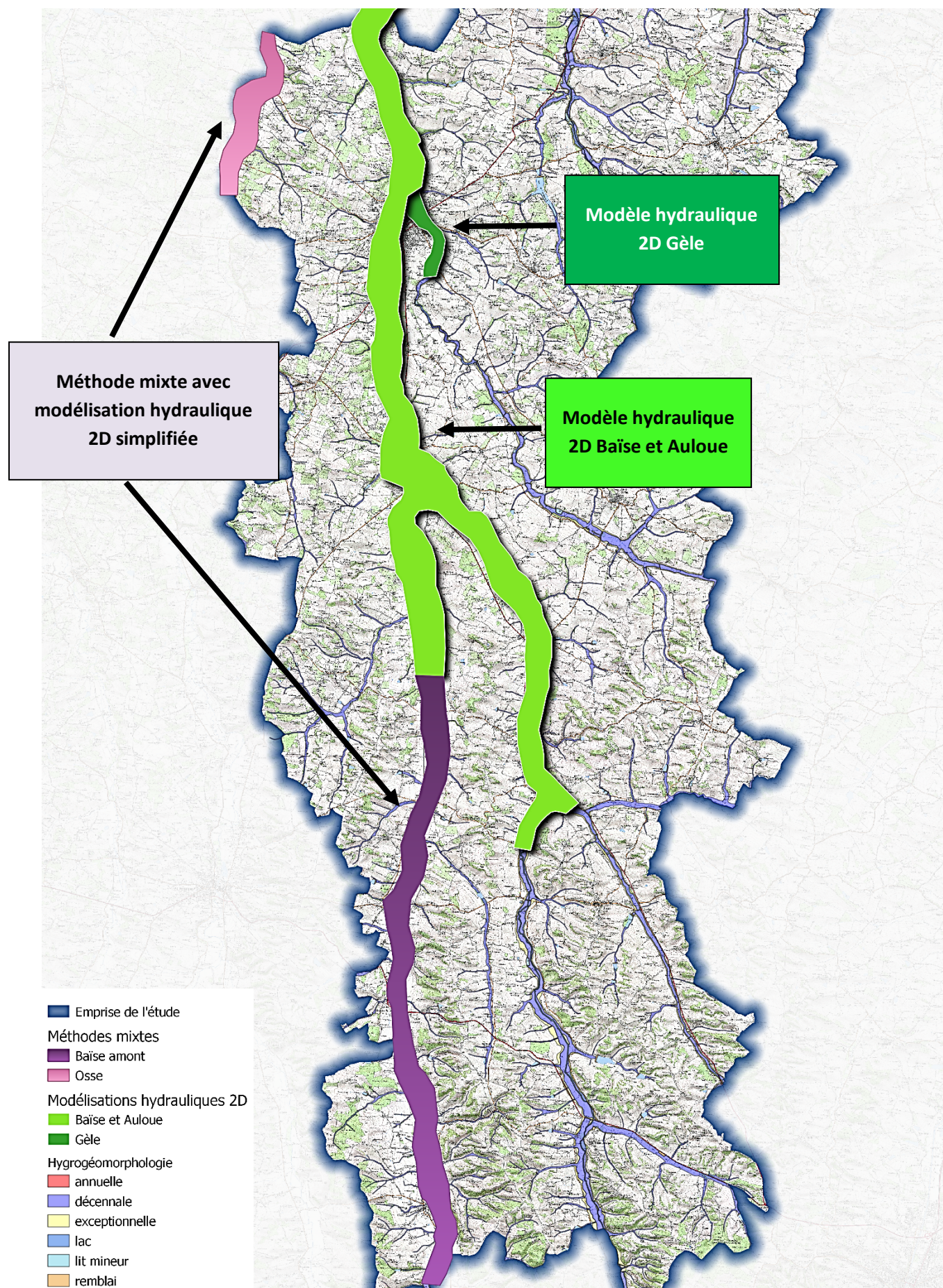
Figure 8 : Emprise des zones modélisées en 2D (détaillées et simplifiées)
