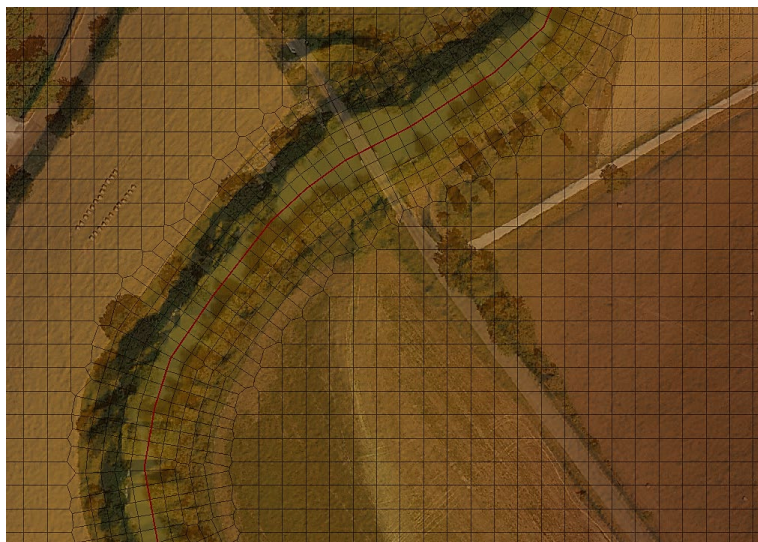
Maillage affiné dans le lit mineur / mailles orientées selon le flux de l'écoulement
