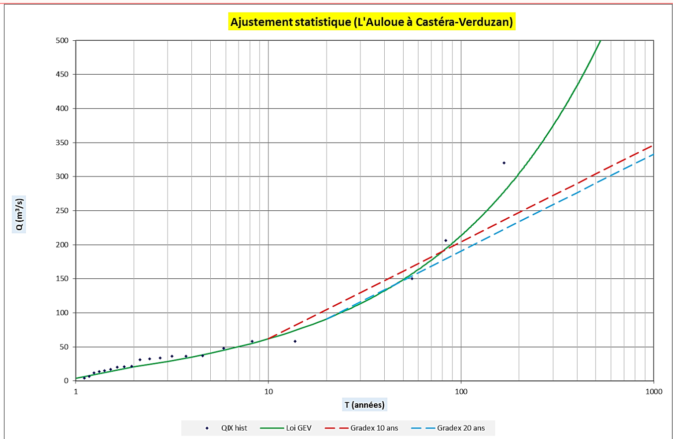
Figure 7 : Analyse fréquentielle des débits de crue pour l'Auloue à Castéra-Verduzan
